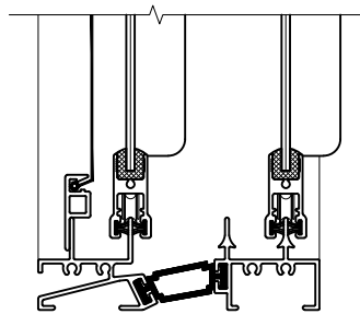
250 SIDESLIDE
