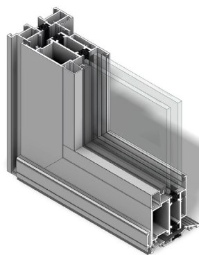
accessABLE™ sill
